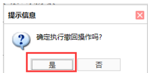
图 1-1-9 提示
