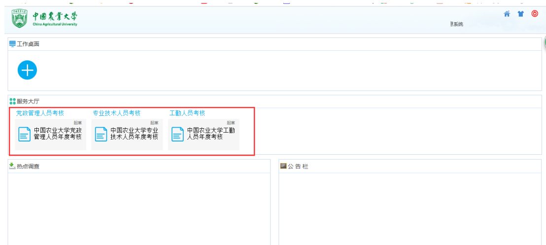
图 1-1-3 表格界面
