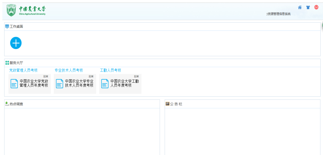
图 1-1-2 主界面
